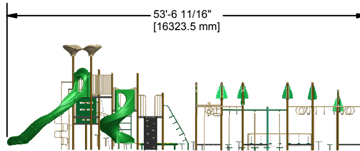
ELEVATION ÉLÉVATION
